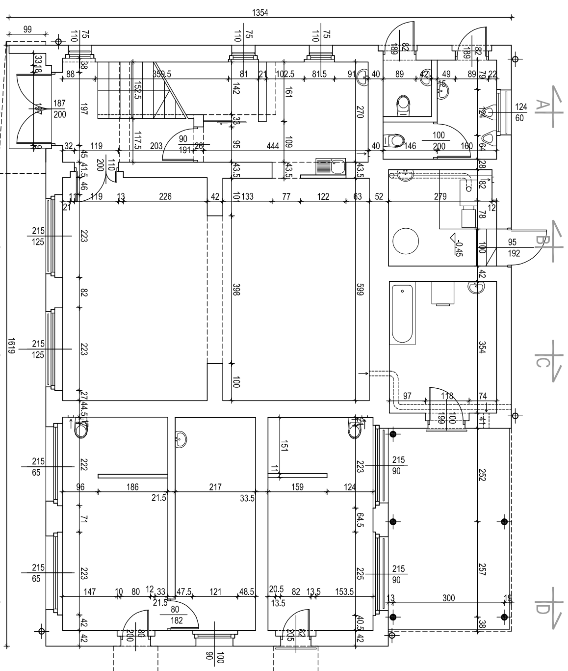
RZUT PARTERU POZ. ±0,00 - STAN ISTNIEJĄCY
