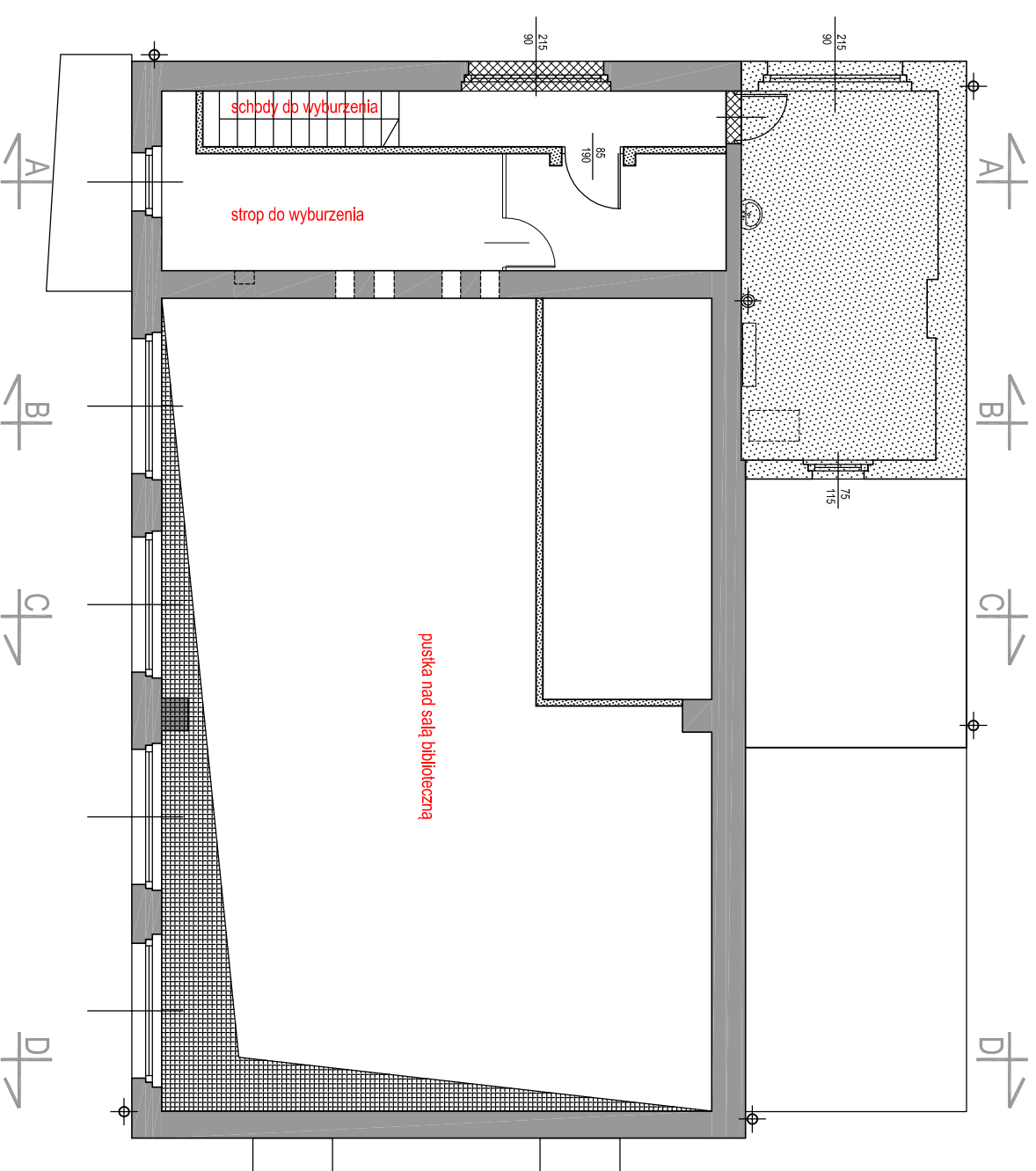
RZUT II PIĘTRA - WYBURZENIA I ZAMUROWANIA
