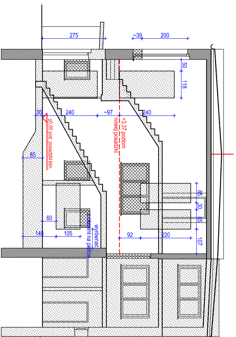
PRZEKRÓJ A - A - WYBURZENIA I ZAMUROWANIA
