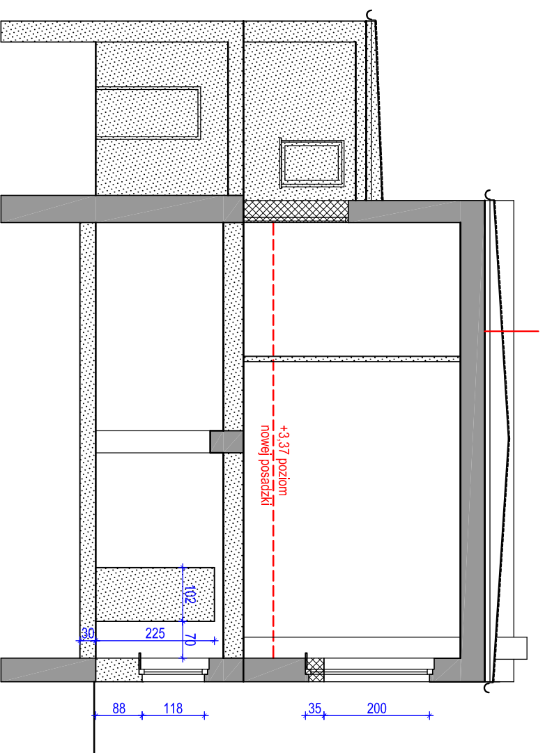
PRZEKRÓJ C - C - WYBURZENIA I ZAMUROWANIA
