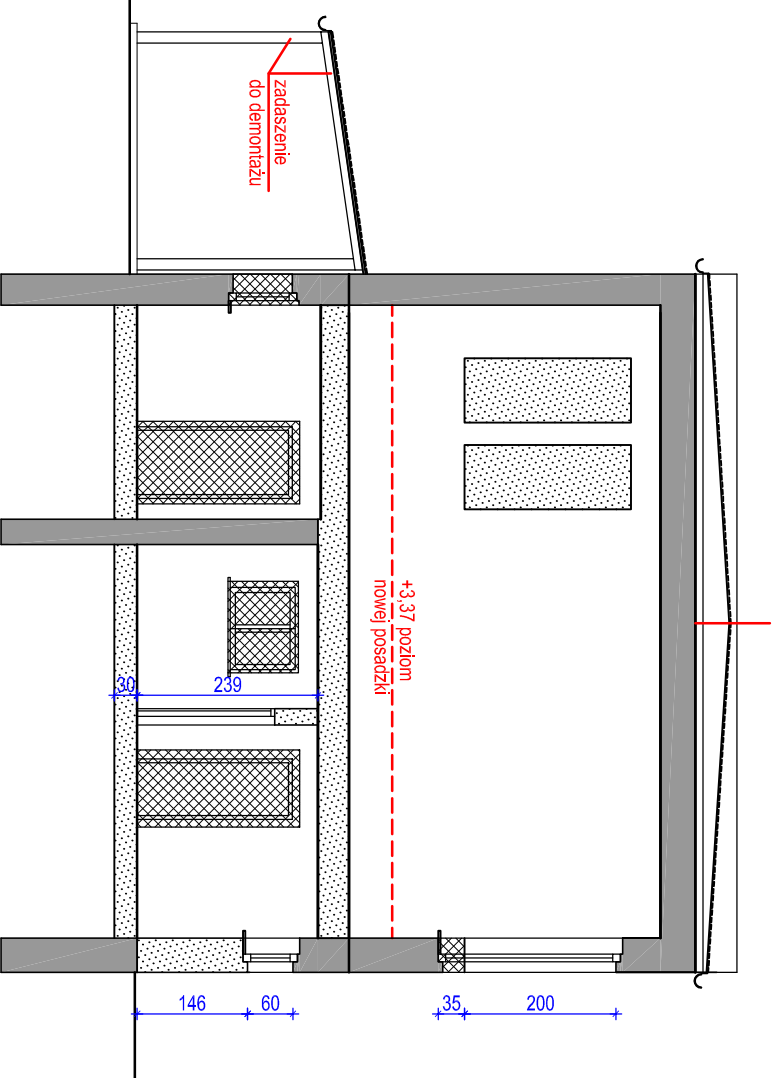
PRZEKRÓJ D - D - WYBURZENIA I ZAMUROWANIA
