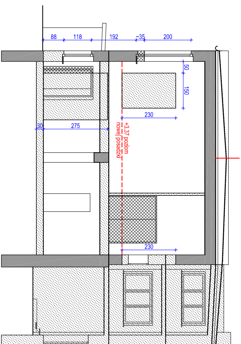
PRZEKRÓJ B - B - WYBURZENIA I ZAMUROWANIA
