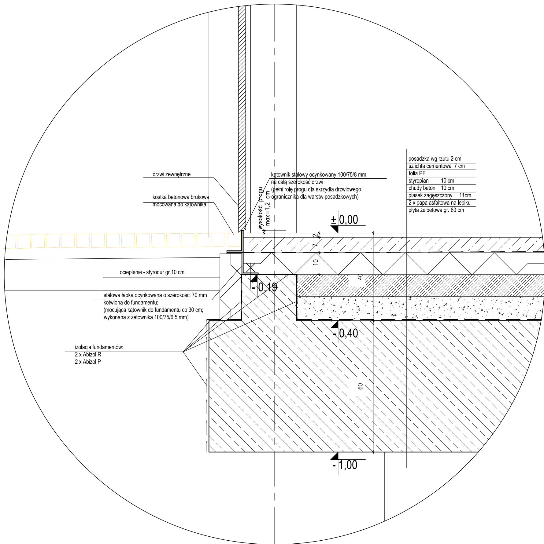
DETAL A - WYJŚCIE Z POM. 1.10, 1.11 (TOALET ZEWNĘTRZNYCH) NA TEREN
