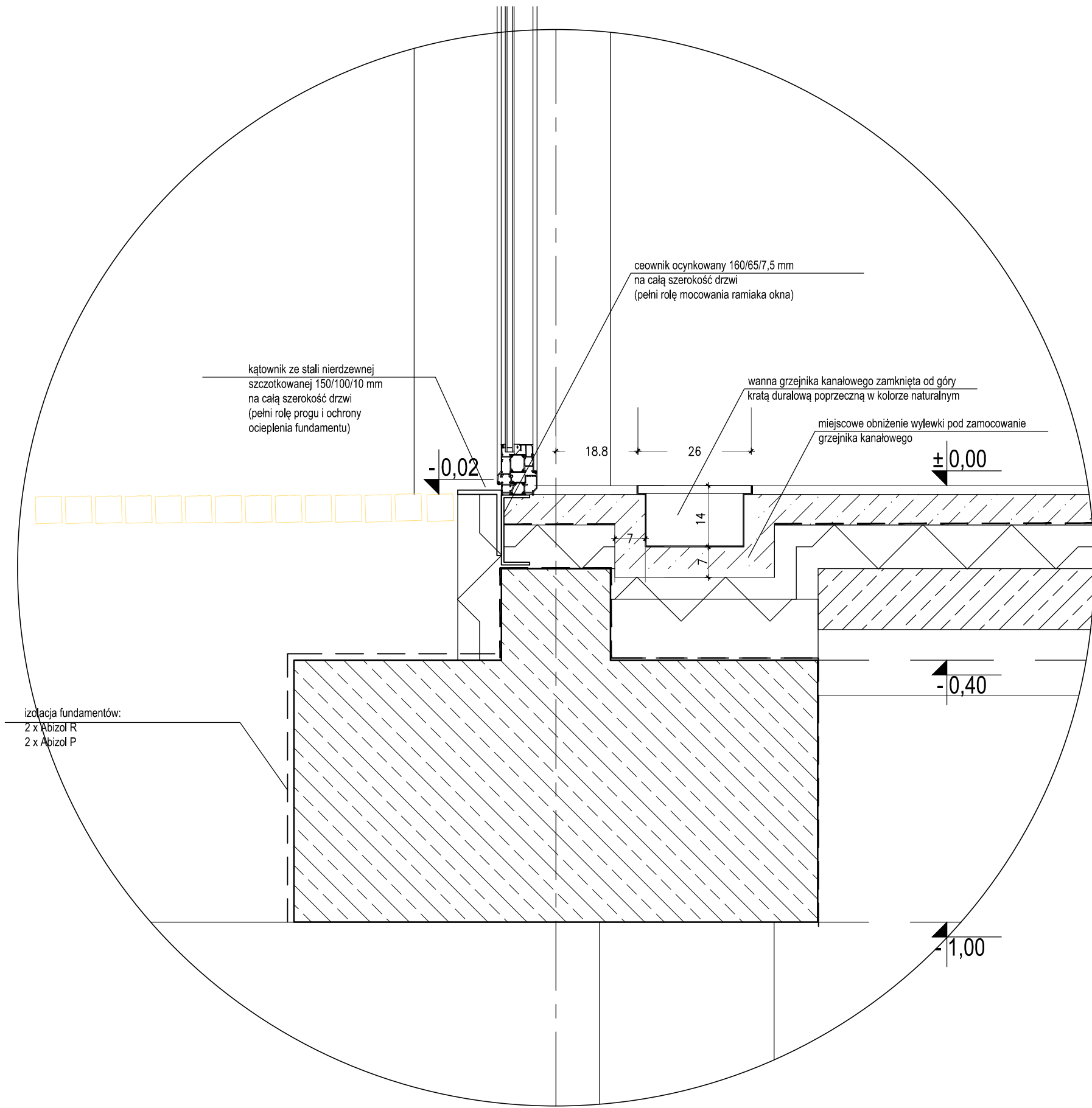
DETAL B - WYJŚCIE Z PO. 1.3 (SALI ODCZYTOWEJ) NA TARAS
