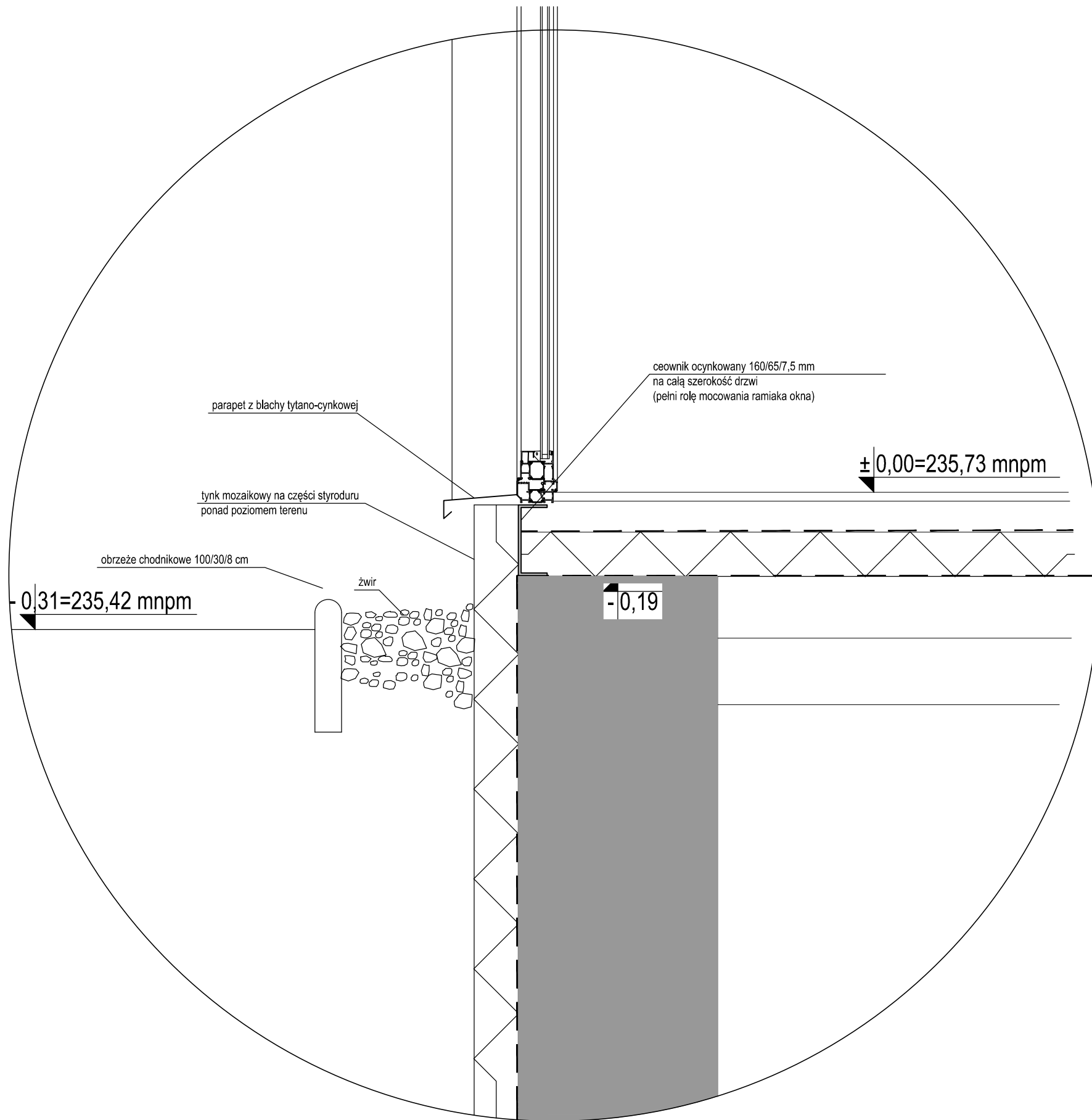
DETAL C - OKNA BALKONOWE POM.1.5 ( POM. DYREKCJI I KSIĘGOWOŚCI)
