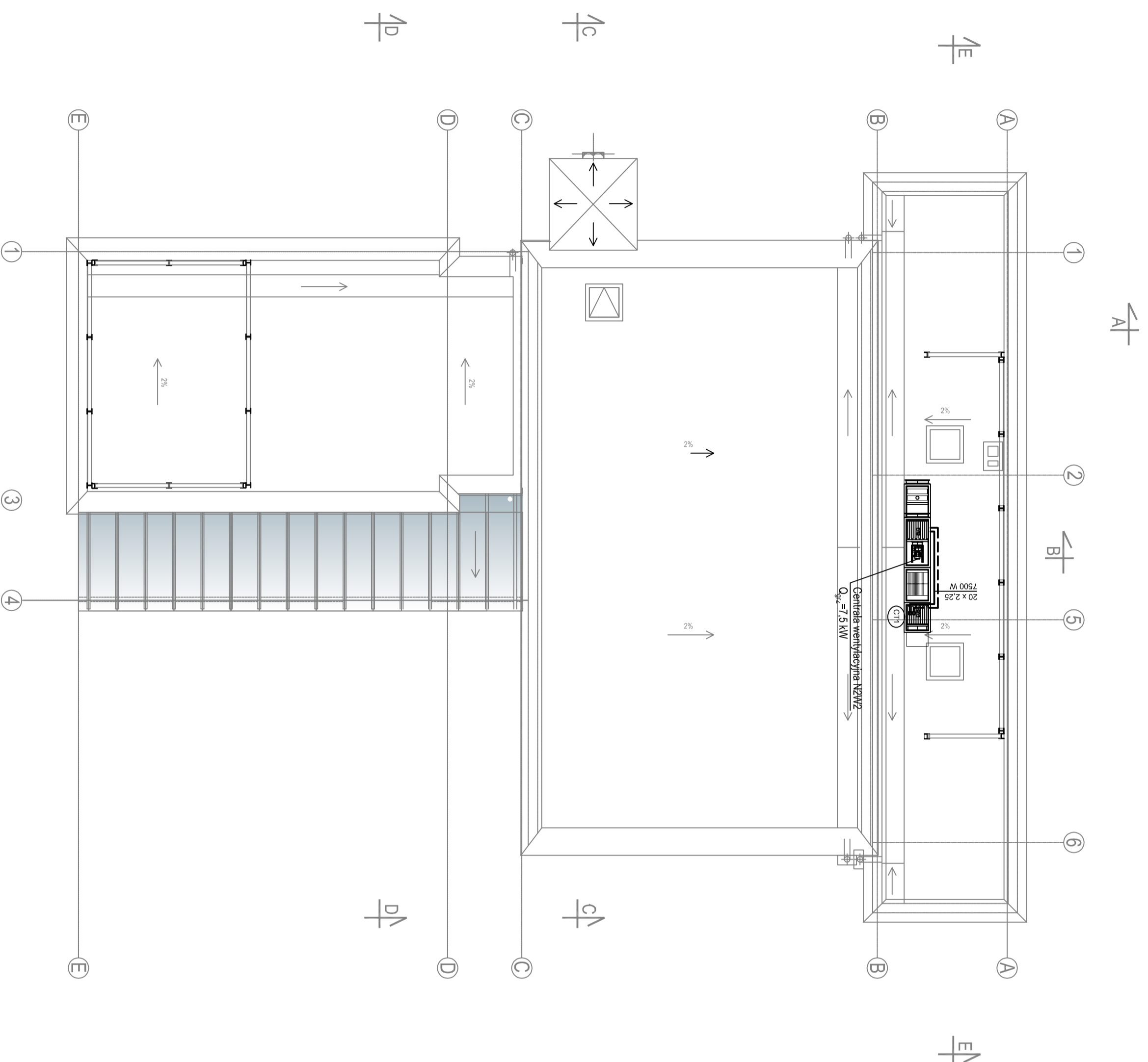
RZUT DACHU
